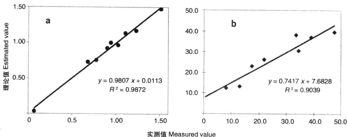
图 2 大气污染物实测值与生物监测指标评价体系理论推导值的线性拟合
