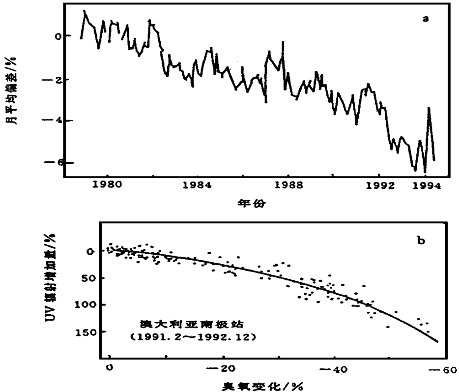
图1 臭氧浓度的变化及UV辐射的关系 (USGCRP, 1995)
