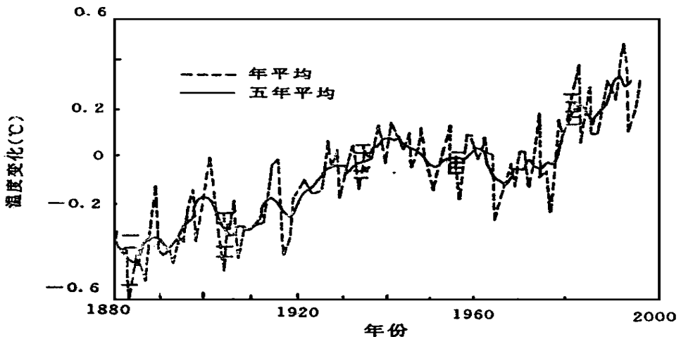
图 2 过去 100 a 全球平均温度的变化 (据 Hansen, 1995)
