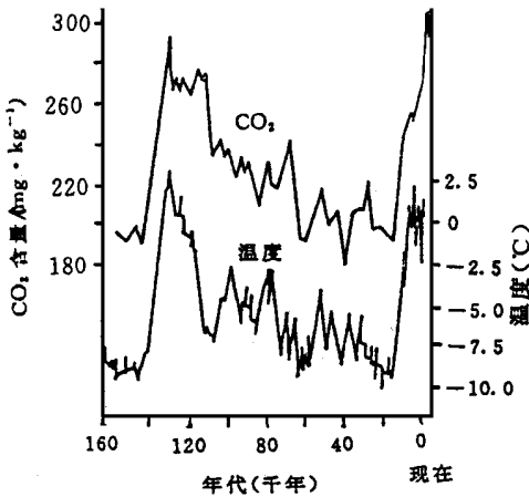
图3 大气中CO 2 增加的状况及趋势 [9]
